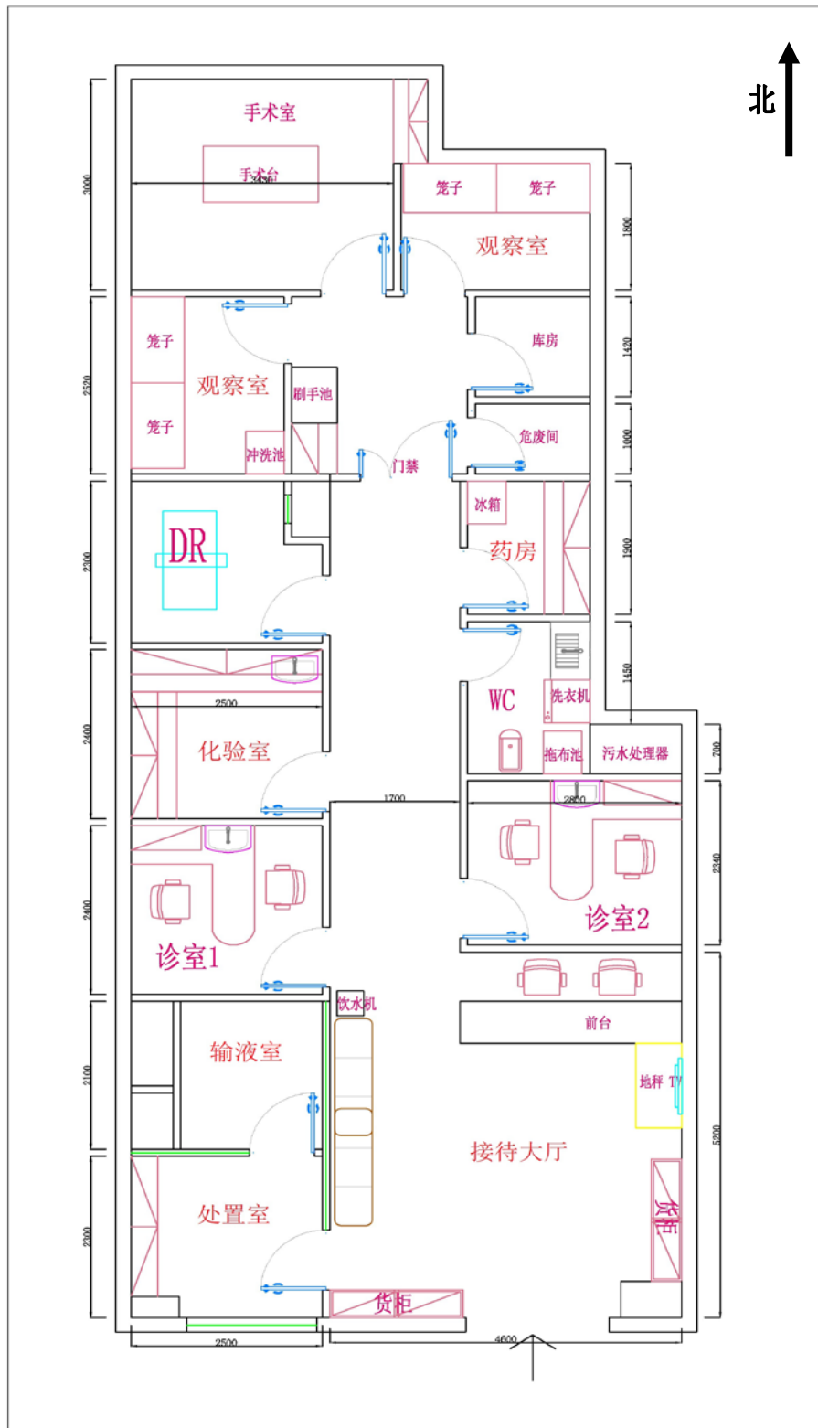
图3 项目平面布置图（1:100）
