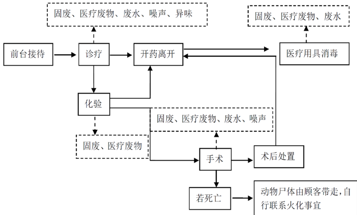
图5 项目营运期工艺流程和产污环节示意图
